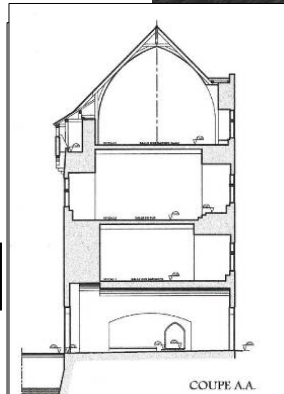
Vues en plan, coupe et façade sur Autocad
